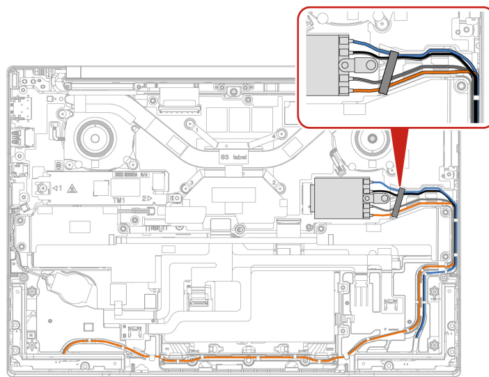
Тип 3: модуль беспроводной сети WAN 5G
