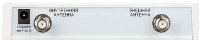
Рисунок 2. Тыльная панель усилителя
