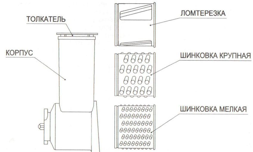
Рисунок 2 - Порядок сборки приставки-овощерезки.
