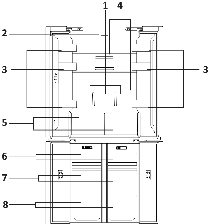
Схема устройства
