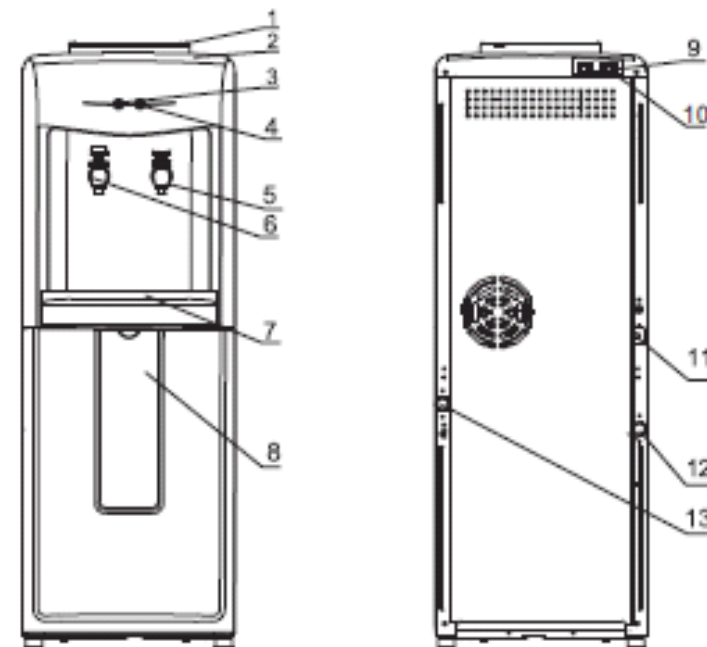
Рис.1 Схема аппарата V118 E
