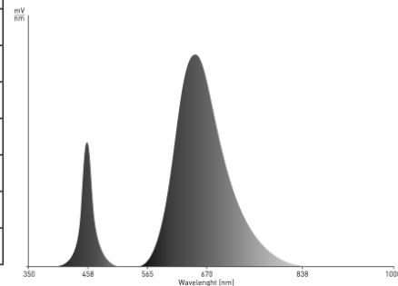
СПЕКТРОГРАММА ИЗЛУЧЕНИЯ
