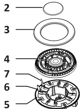
WOK-конфорка
