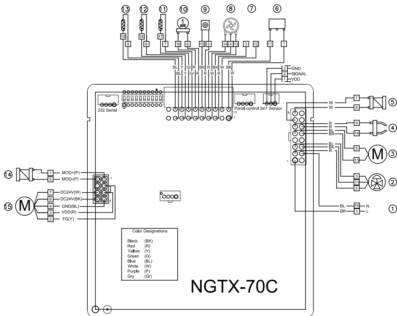
Рисунок 16. Схема электрическая.
