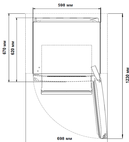
Մատնարանային սարքի աշխատանքային չափերը Муздаткыч өлчөмдөрү
