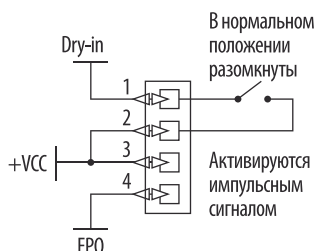
Вход “Сухие контакты”
