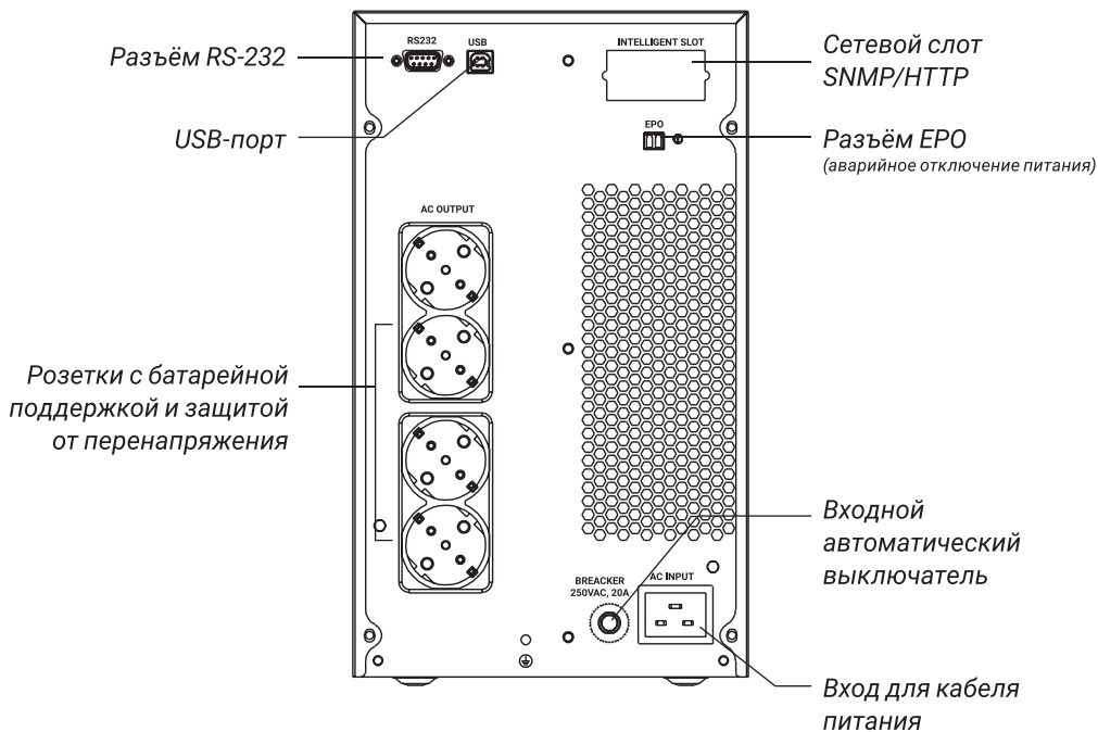
ИБП Na+ TAE 3000
