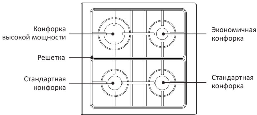
Расположение конфорки в модели M16-1
