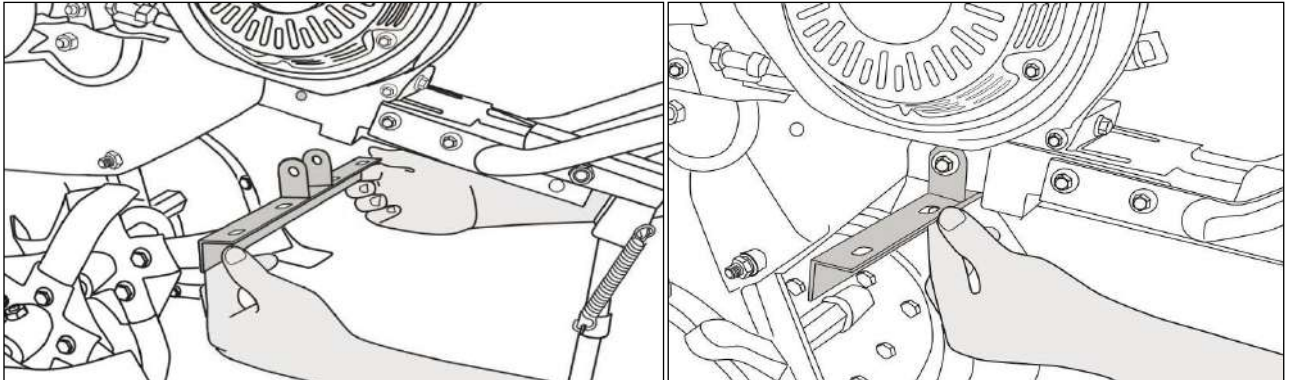
Рис. 10-11. Установка передней балки крепления крыльев
