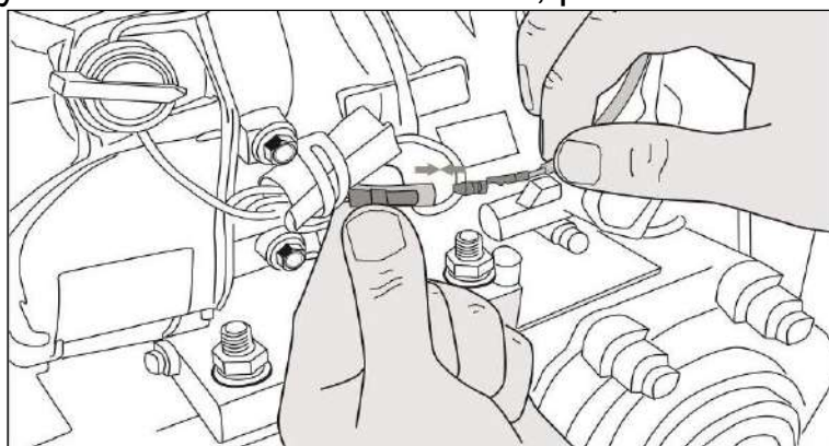
Рис. 4. Соединение клеммы выносной кнопки стартера
