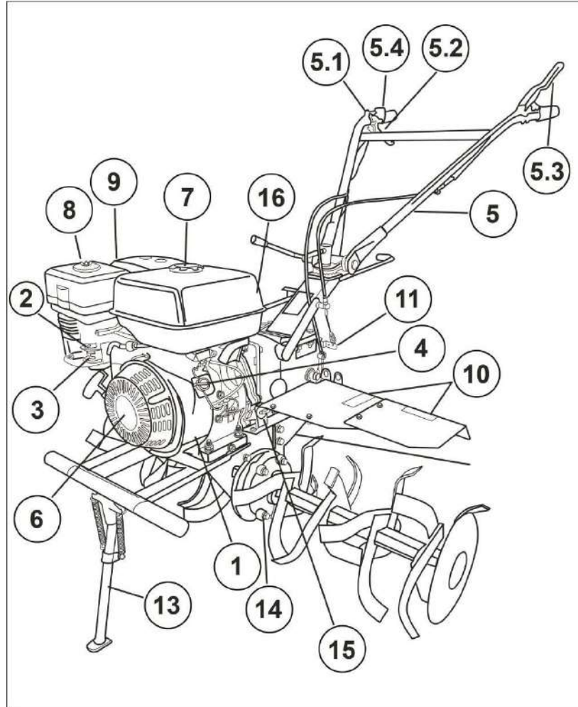
Рис. 1. Общий вид
