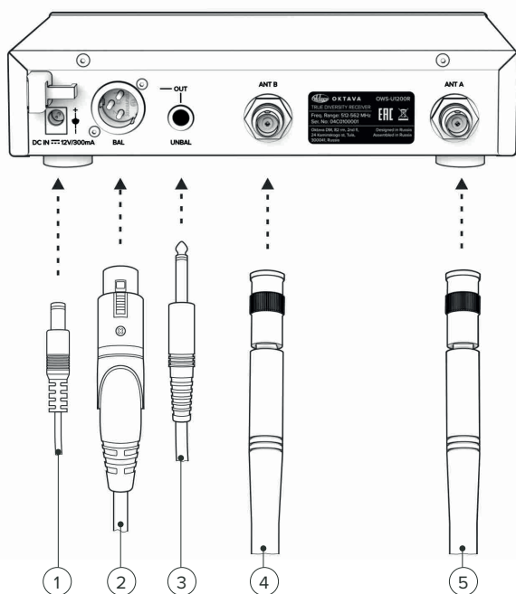
Схема 1. (1. Питание, 2. XLR, 3. Jack , 4-5. Антенны.)
