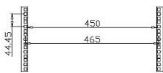
установочные размеры
