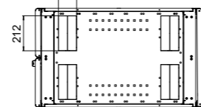
Вид снизу
